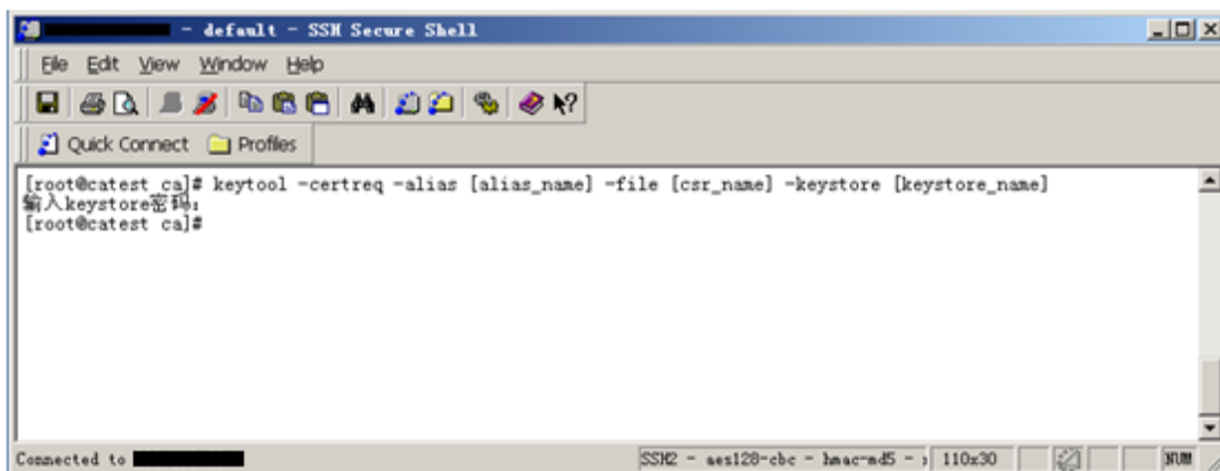
图表二 生成 csr 文件
